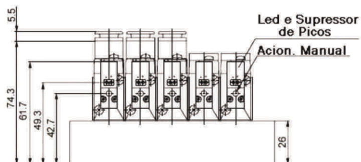
Conector DIN
