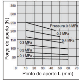
F. Externa CHS3-63D F. Interna
