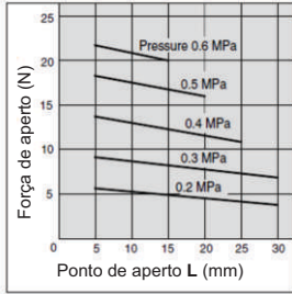
F. Externa CHS3-20D F. Interna
