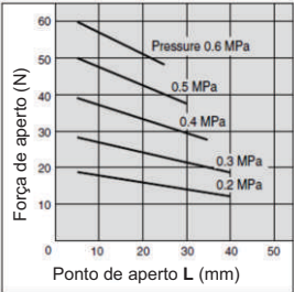
F. Externa CHS3-32D F. Interna
