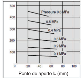
F. Externa CHS3-80D F. Interna
