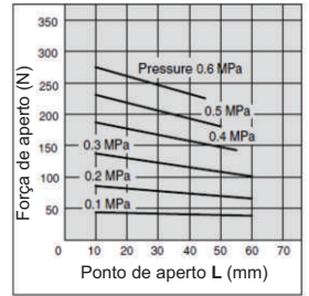
F. Externa CHS3-63D F. Interna
