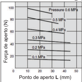
F. Externa CHS3-40D F. Interna
